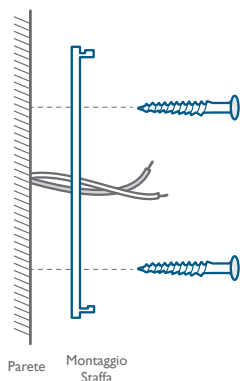
Senza cuneo di montaggio da 15°
