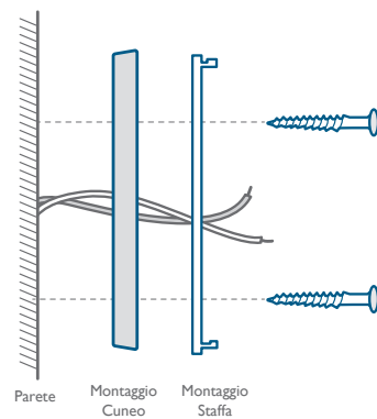
Con cuneo di montaggio da 15°
