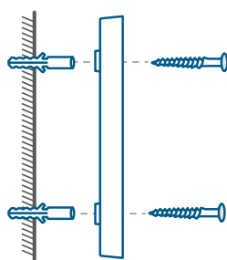
Montáž Držák
