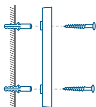
取り付けマウント
